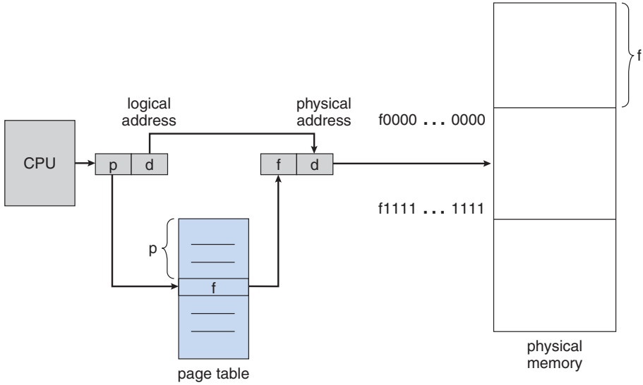
Figure 7.10 Paging hardware.
